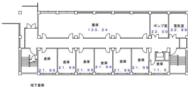
1階（457.30m 2 ）
