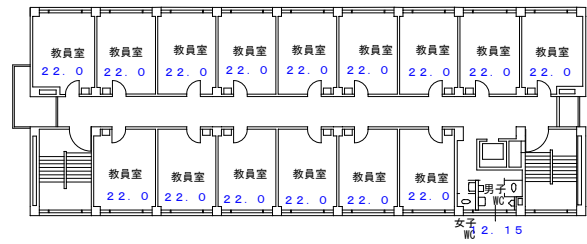
7階（465.97m 2 ） 1 : 500
