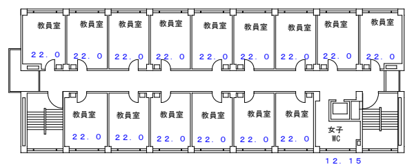
4階（465.97m 2 ）
